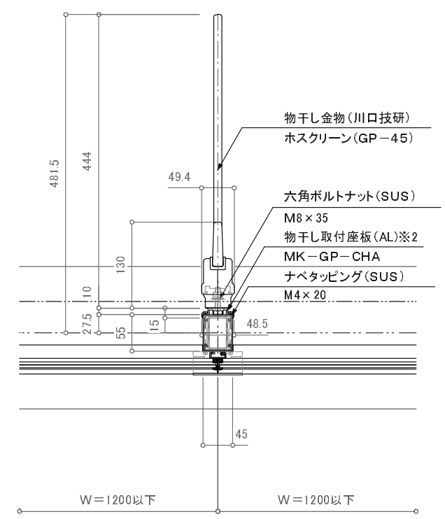
物干し金物部平面詳細図
