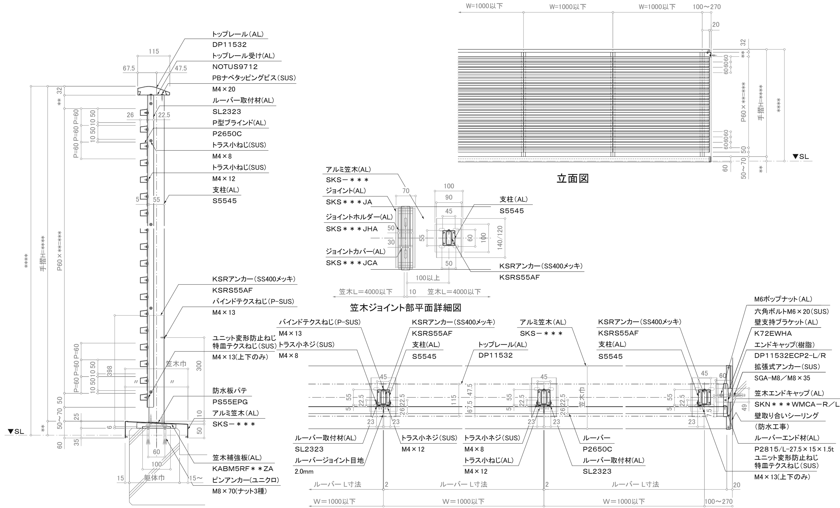
断面図
