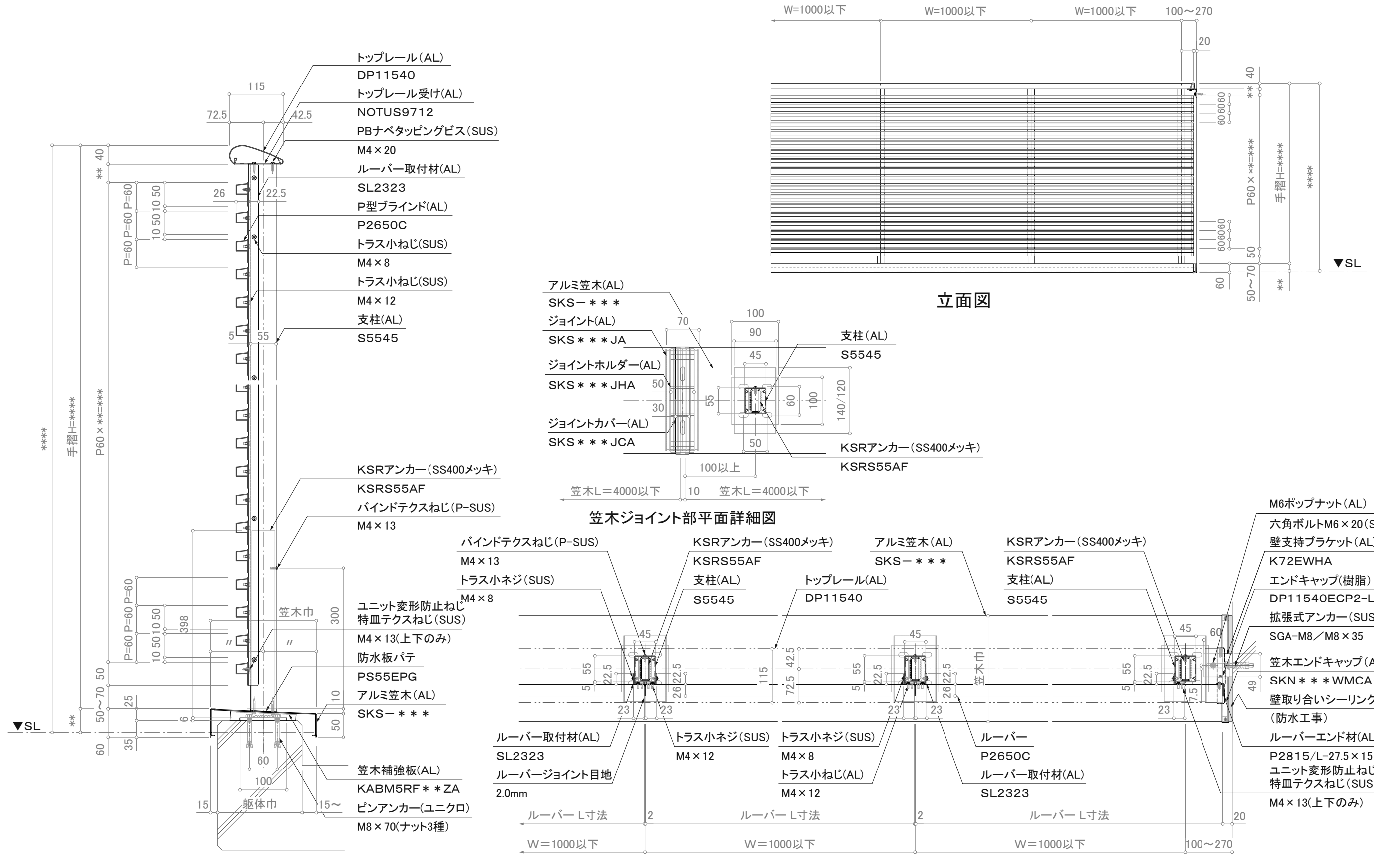
平面詳細図
