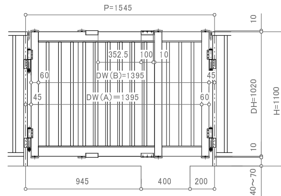
ストローク300の場合の参考立面図(±0)
