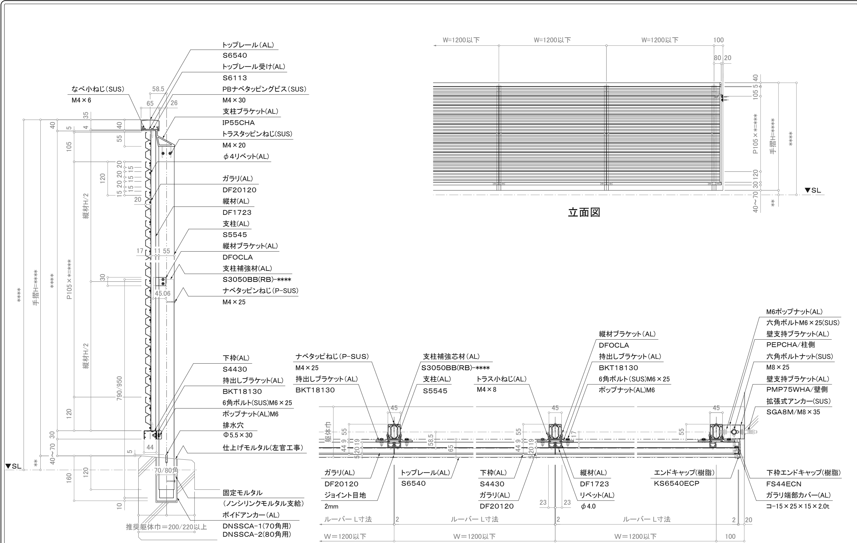
断面図
