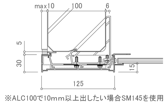
SM125(ALC用Max)
