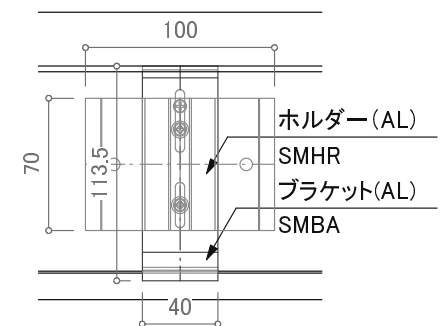
RC用ホルダー
