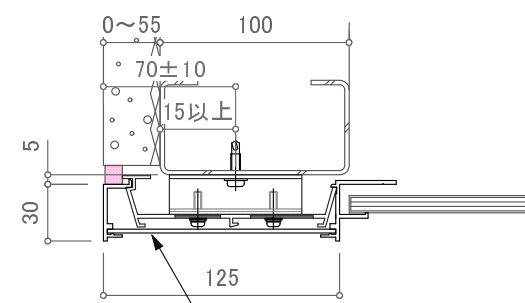
SM125R(鉄骨用)
