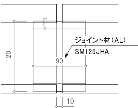
ジョイント部詳細
