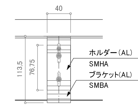
ALC用ホルダー
